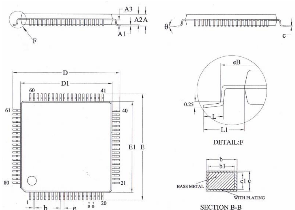
图 86 LQFP80 封装图
