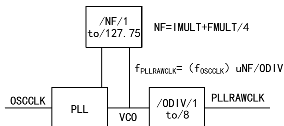
图 20 系统 PLL
