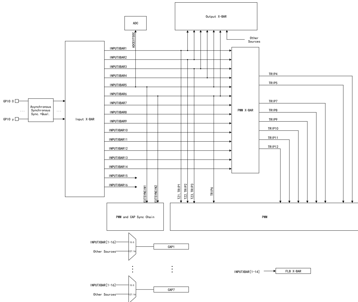
图 5 输入 X-BAR
