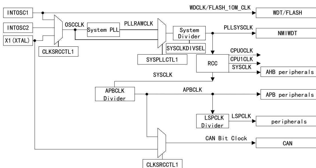
图 20 系统 PLL
