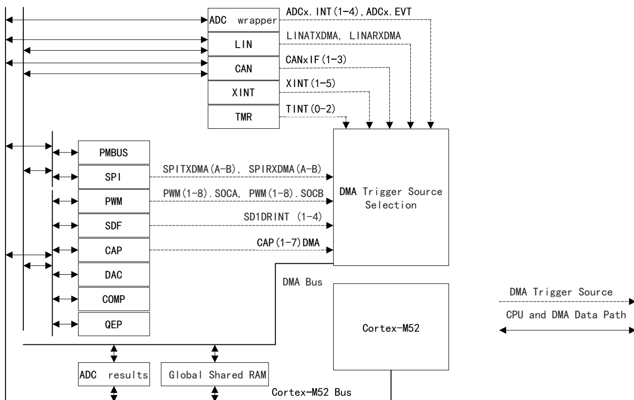
图 9 DMA 结构框图
