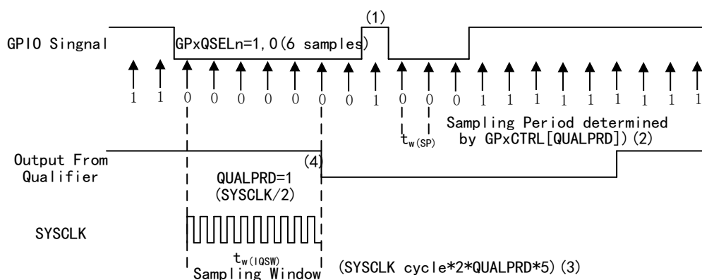
图 31 采样模式
