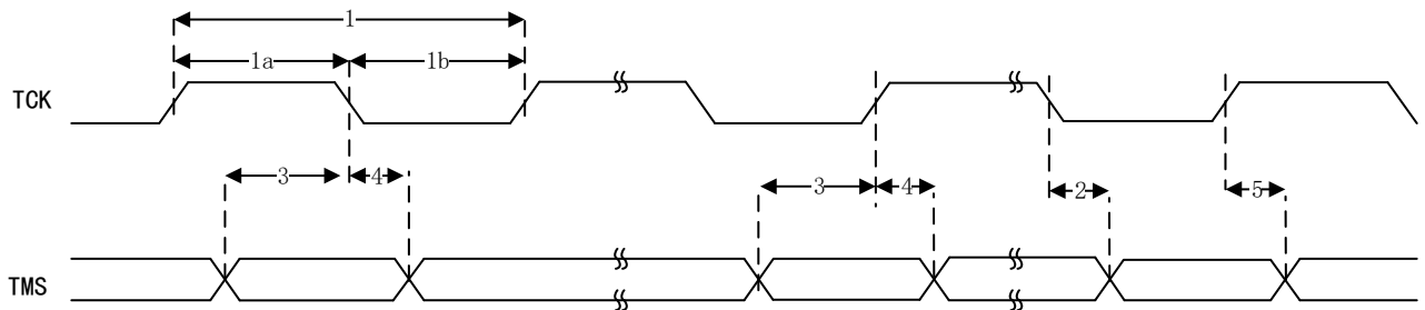
图 29 cJTAG 时序图
