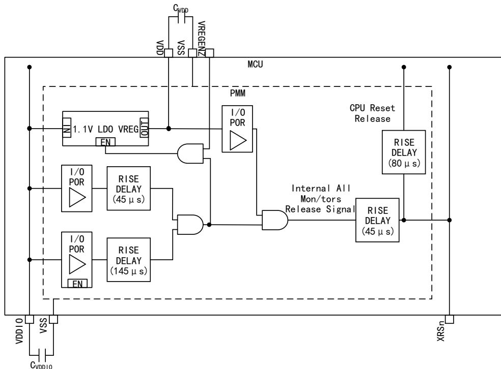
图 13 PMM 结构框图
