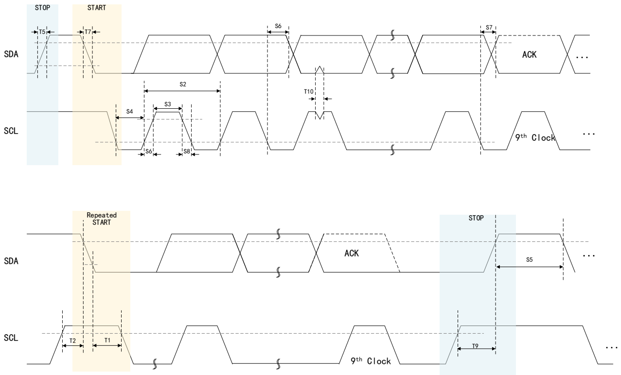
图 70 I2C 时序图
