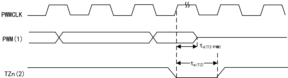
图 63 PWM Hi-Z 特征
